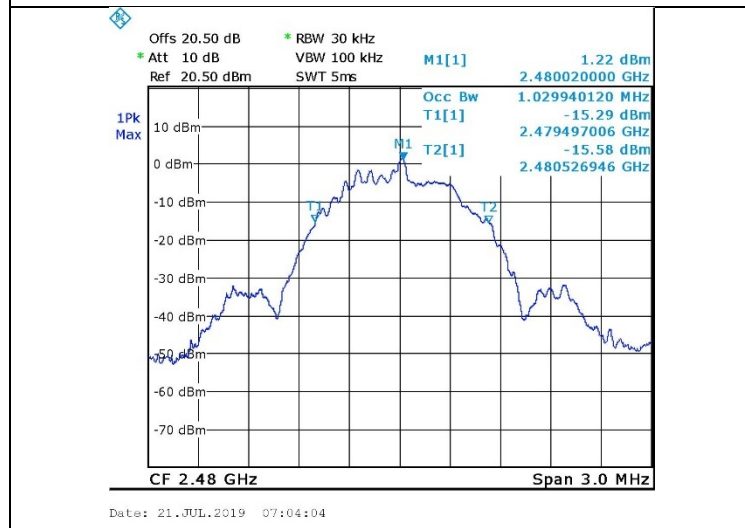
Figure 33. 2480.0 MHz, BLE
