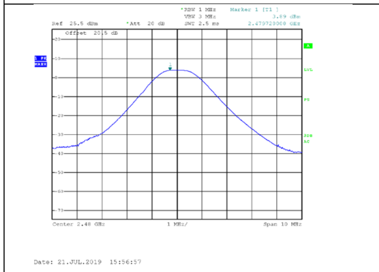
Figure 19. 2480.0 MHz, BLE
