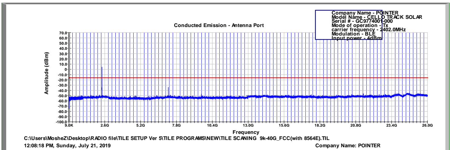
Figure 35 2402.0 MHz, BLE
