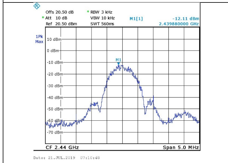
Figure 27. 2440.0 MHz, BLE
