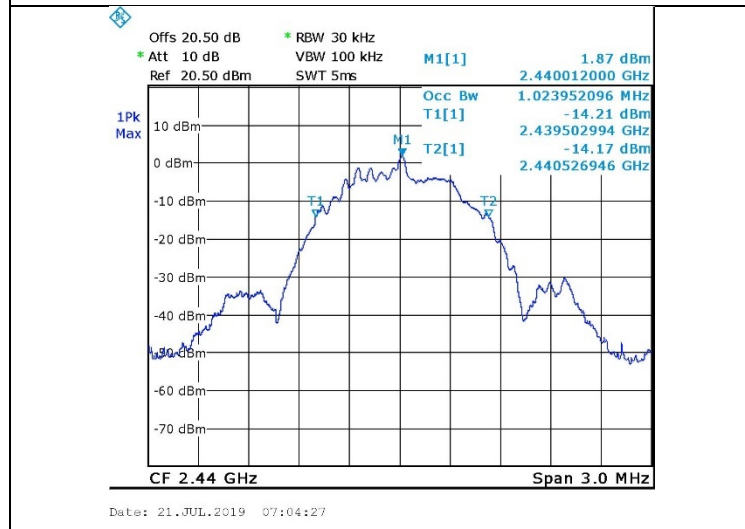
Figure 32. 2440.0 MHz, BLE
