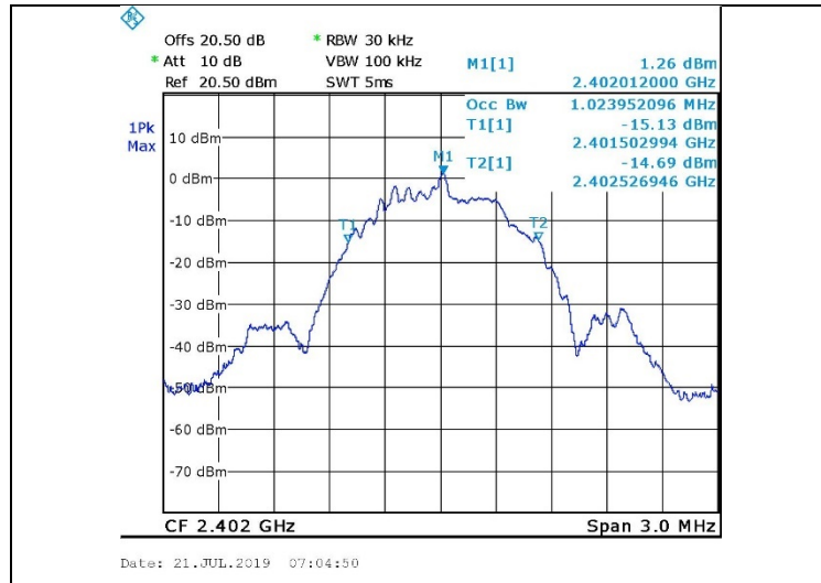
Figure 31. 2402.0 MHz, BLE
