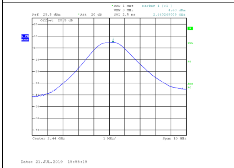
Figure 18. 2440.0 MHz, BLE
